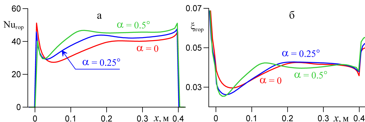
Рис. 8. Распределение числа Нуссельта (а) и коэффициента сопротивления (б) по длине при различных углах раскрытия для канала с горячим теплоносителем
