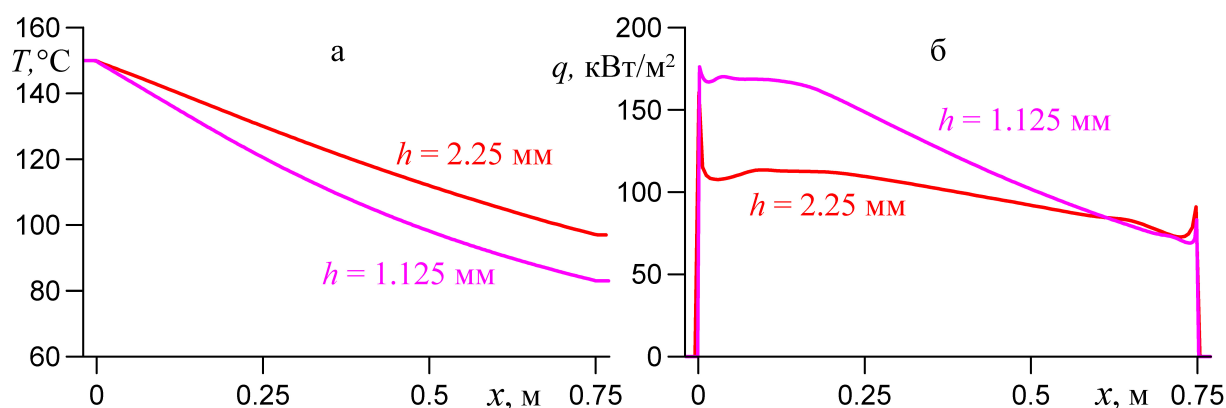
Рис. 5. Изменение средней температуры горячего теплоносителя (а) и теплового потока в стенку (б) по длине канала высотой 2.25 мм и 1.125 мм
