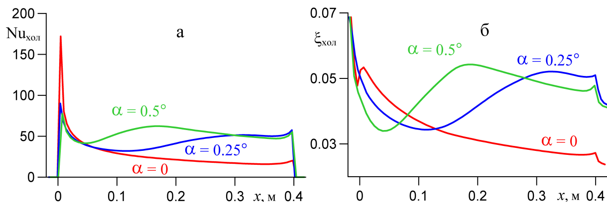
Рис. 9. Распределение числа Нуссельта (а) и коэффициента сопротивления (б) по длине при различных углах раскрытия для канала с холодным теплоносителем
