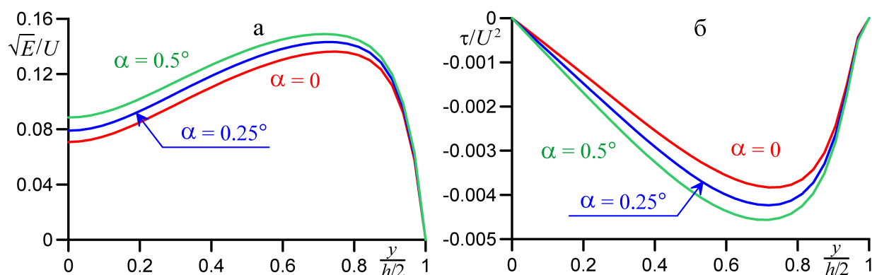
Рис. 10. Распределения по высоте канала интенсивности турбулентности (а) и напряжений Рейнольдса (б) в конце теплообменной части канала горячего теплоносителя
