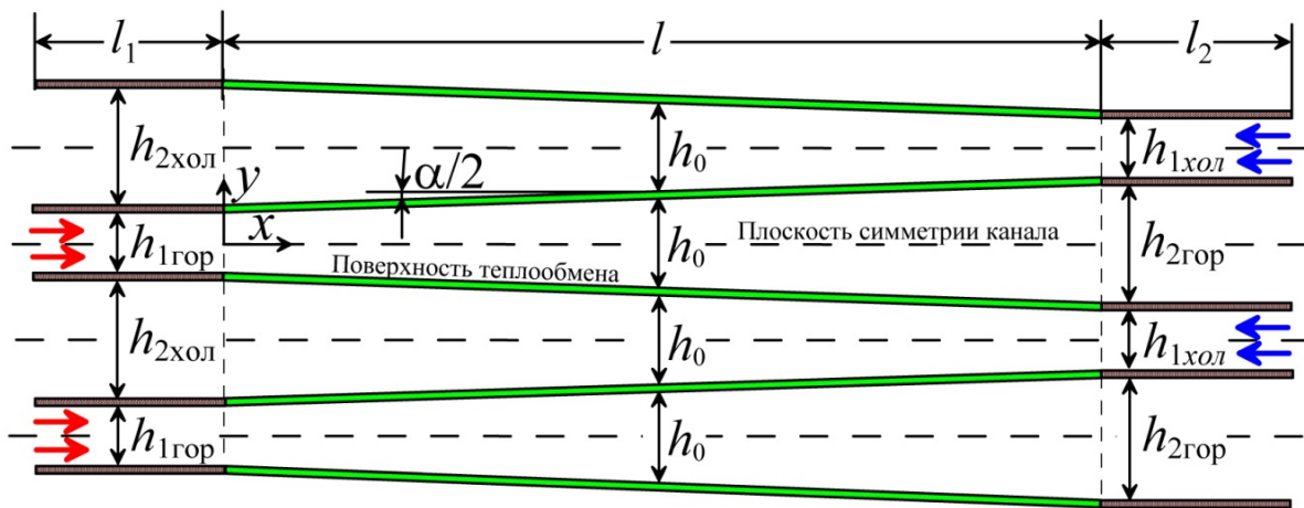
Рис. 1. Расчетная схема плоского противоточного многоканального теплообменника
