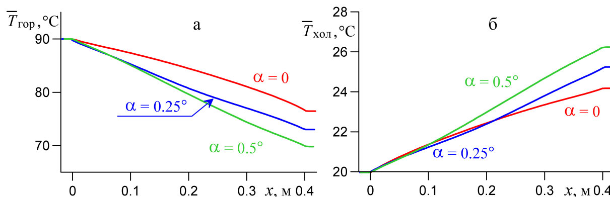
Рис. 7. Распределения по длине средних температур в горячем (а) и холодном (б) каналах при различных углах раскрытия
