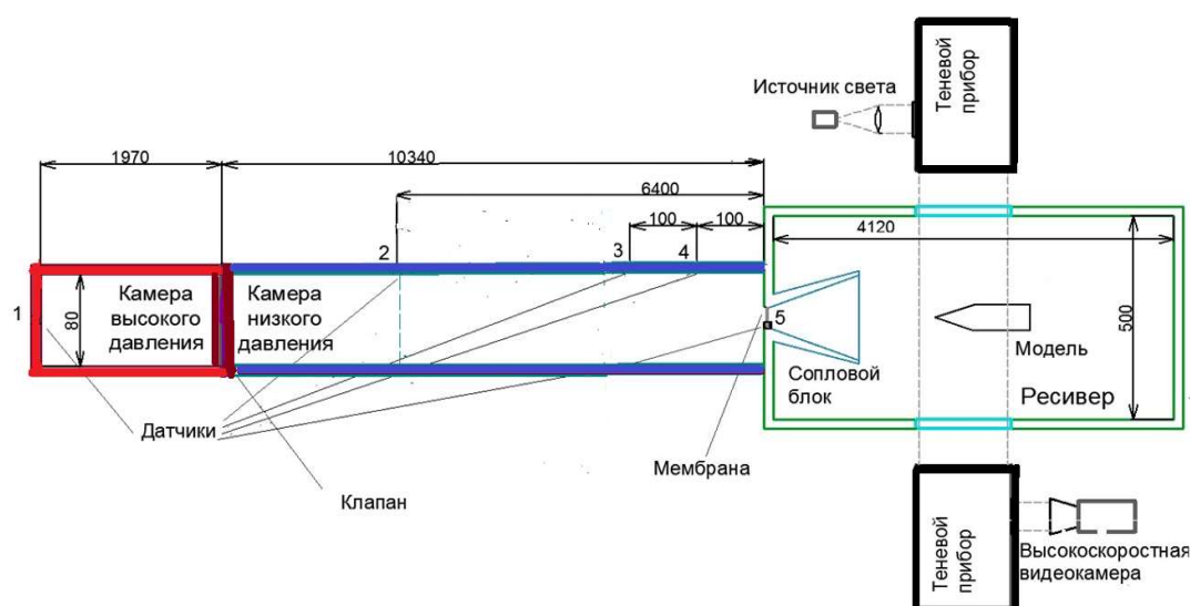
Рис. 2. Схема ГУАТ
