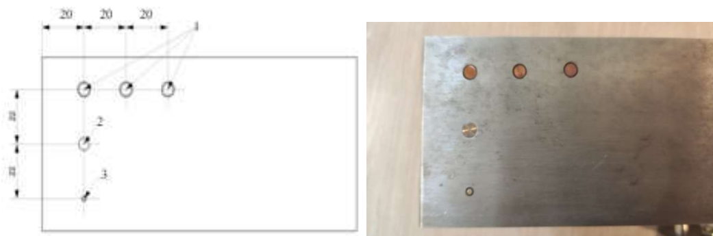
Рис. 5. Эскиз и фото нижней модели с метками установок датчиков: 1 – СТ1, СТ2, СТ3, 2– РСВ, 3 –МСТ
